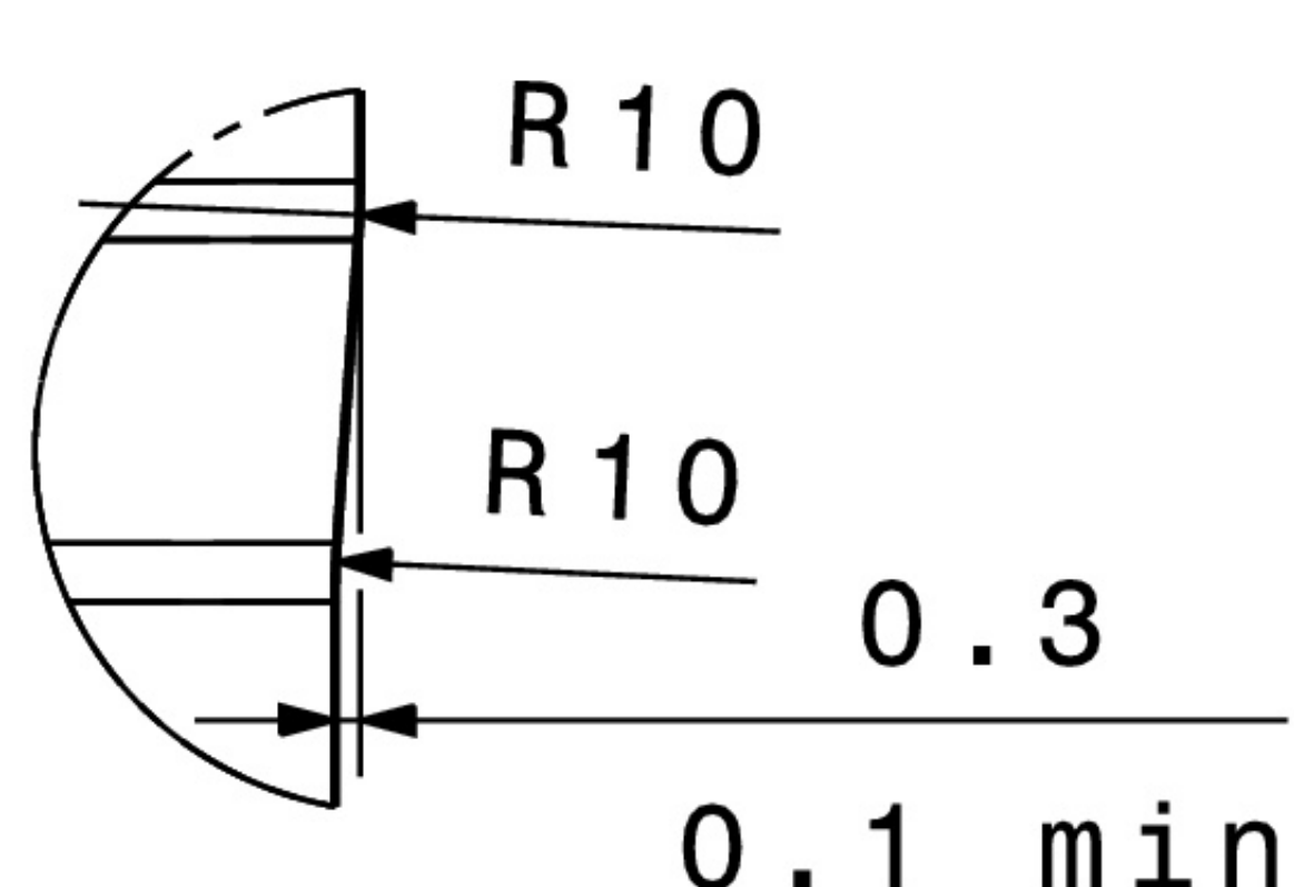
Detail A Maßstab: 3:1
