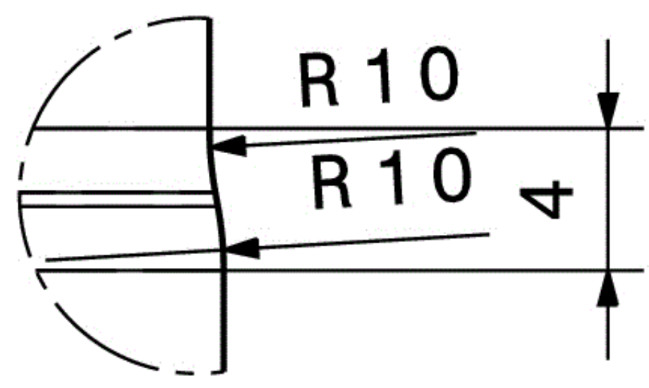
Detail A Maßstab: 2:1
